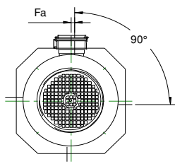
M2AA 160 / 180 M3BP 160 / 180
