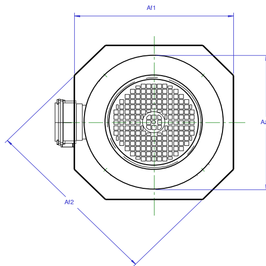
M2AA 160L-180L M2AA 200 - 250
