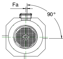
M2AA 160 / 180 M3BP 160 / 180
