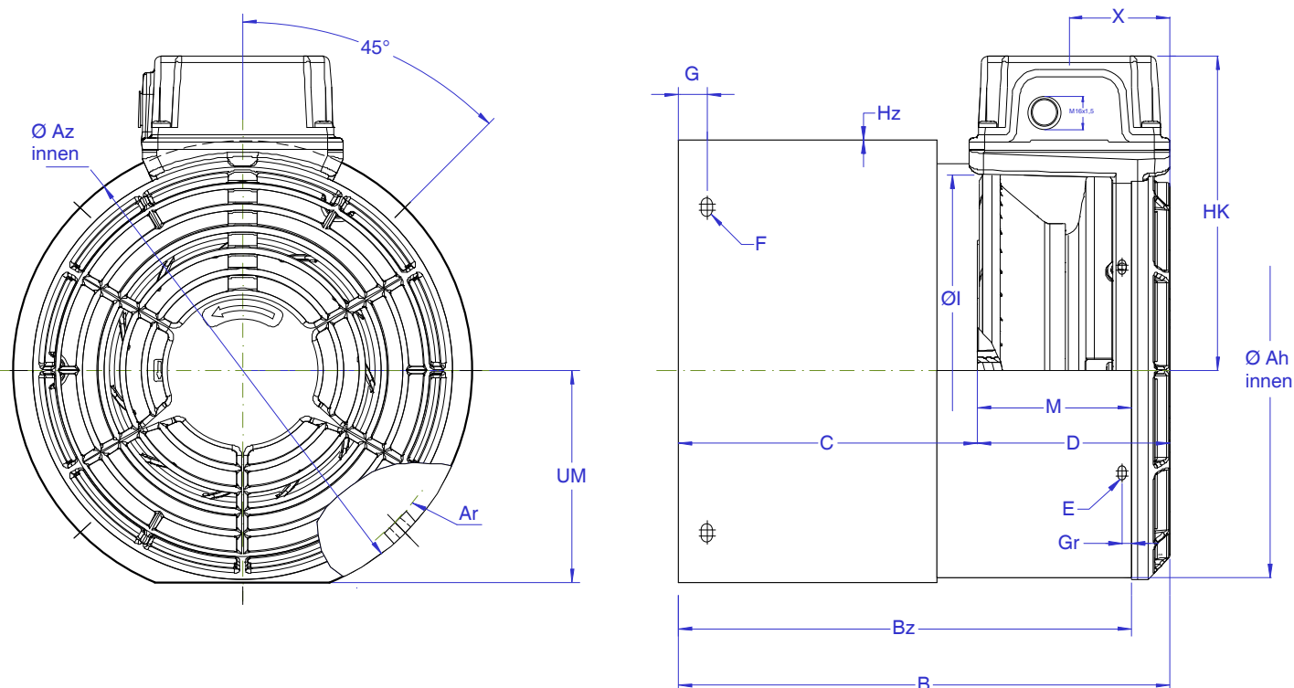
Abmessungen / Dimensions / Côtes / Dimensioni / Cotas
